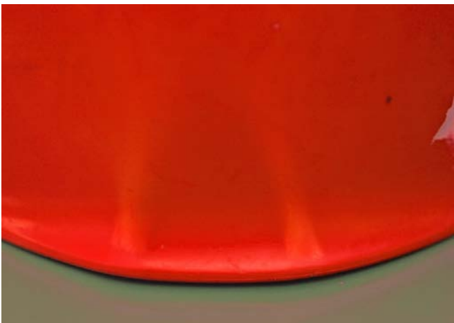
Weißbruchstellen an einem Arbeitsschutz- / Bergsteigerhelm
