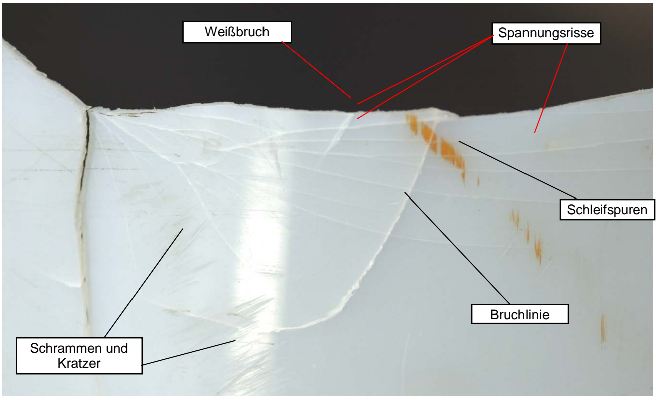
Verschiedene Schadensbilder an einer Trage aus Kunststoff (15 Jahre alt)
